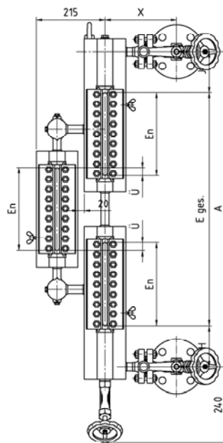
Rechtsmodell
